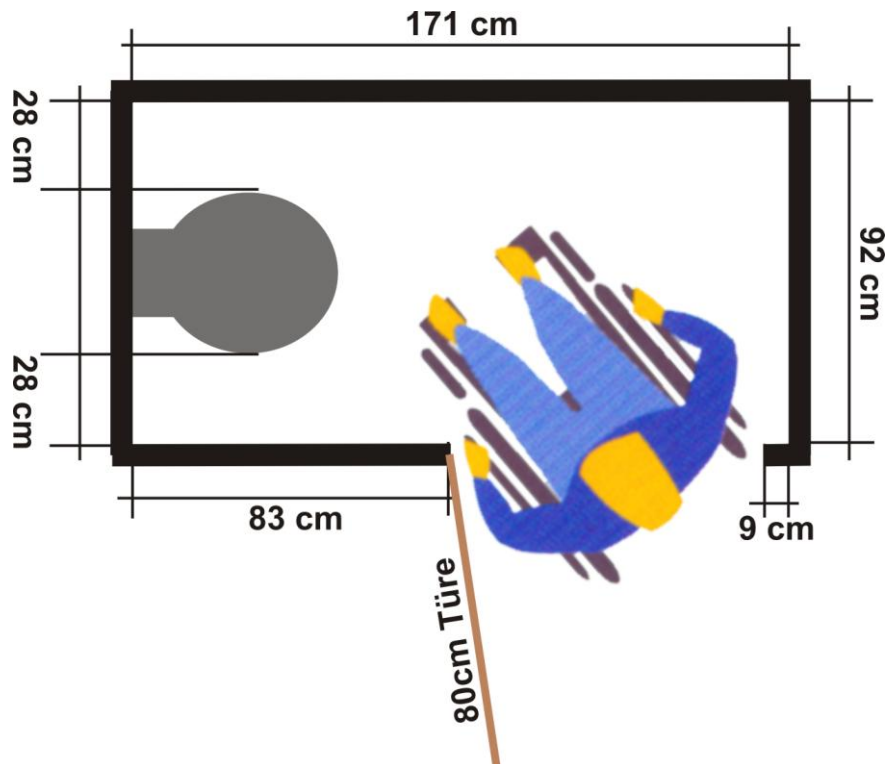
Skizze - Toilette
